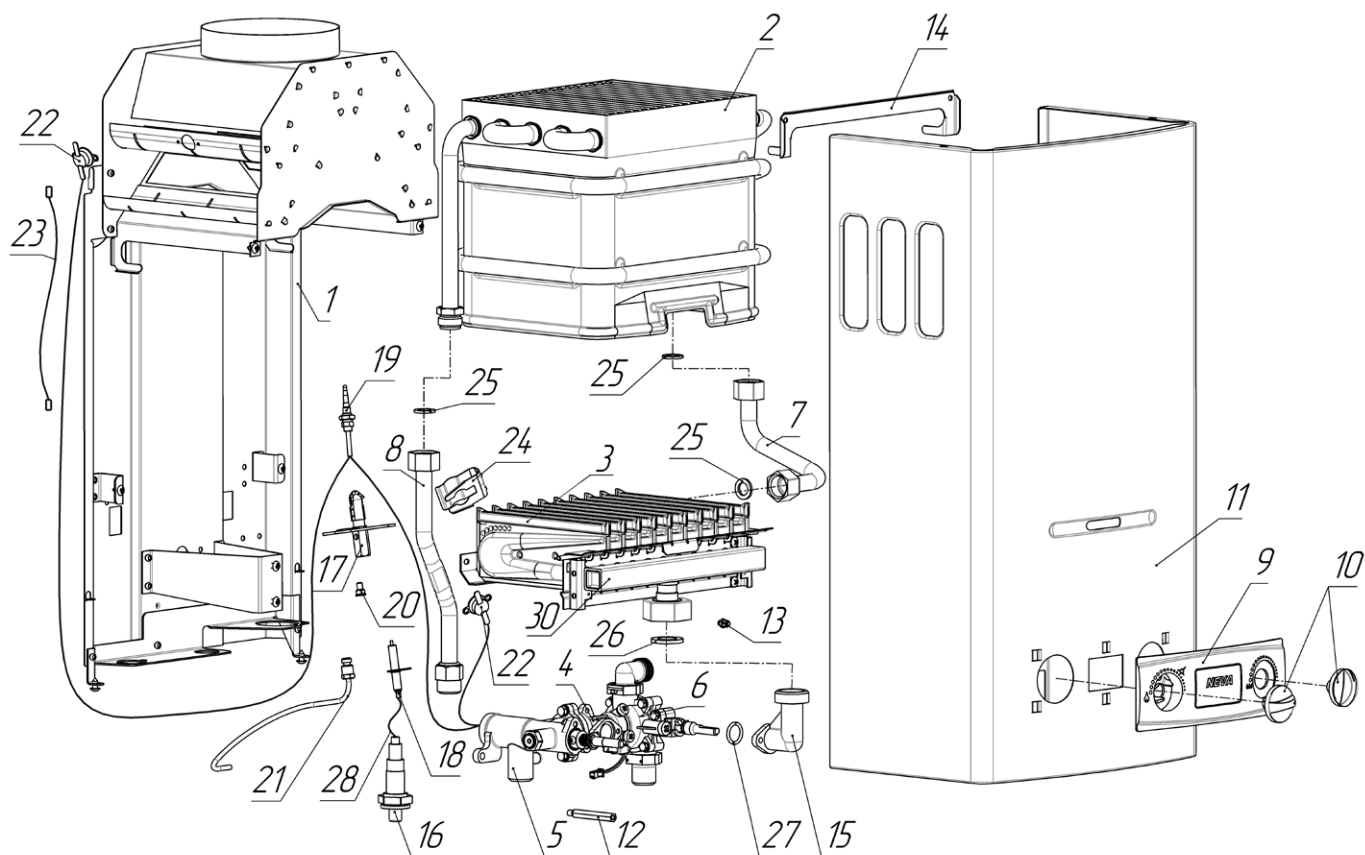
Взрывная схема NEVA 4511 P также подходит для NEVA 4513 P.
