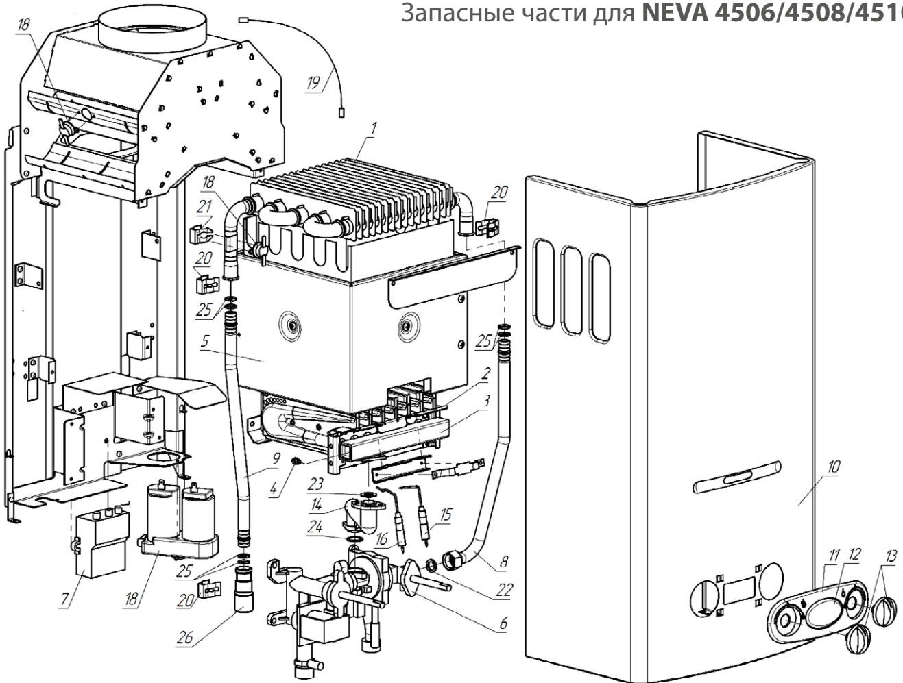
Взрывная схема NEVA 4506 и NEVA 4508.
