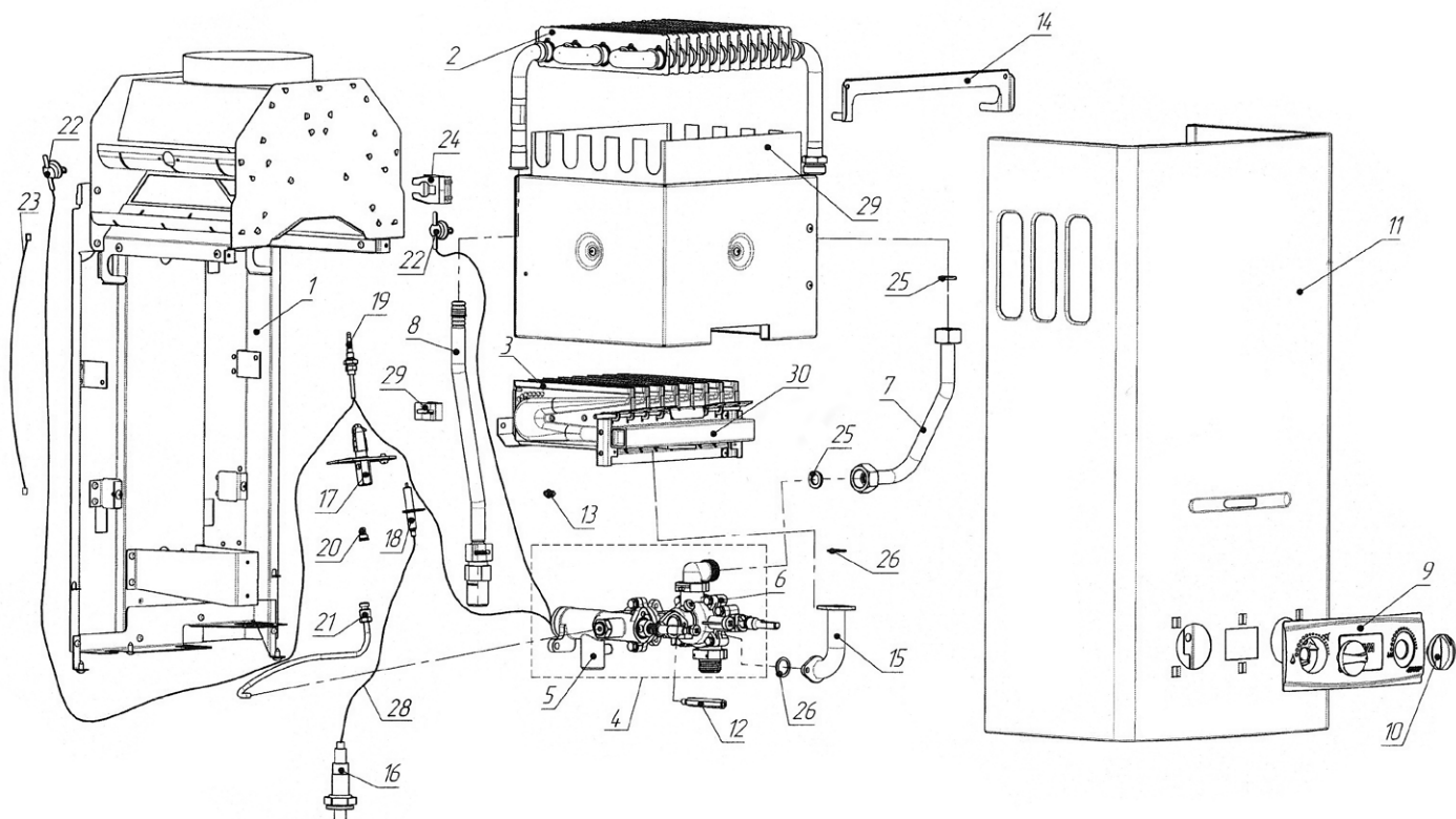
Взрывная схема NEVA 4510 P.
